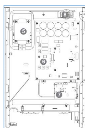
下電控箱-正面
