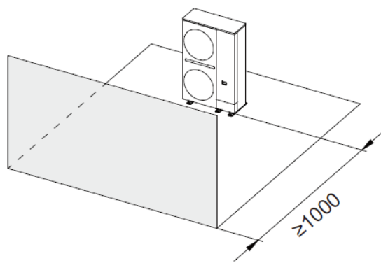
單台室外機
