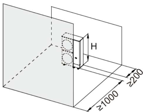
單台室外機
