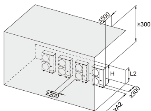
多台室外機
