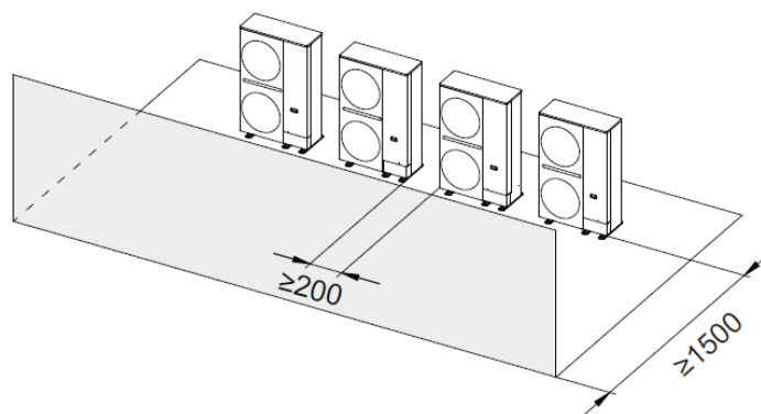
多台室外機
