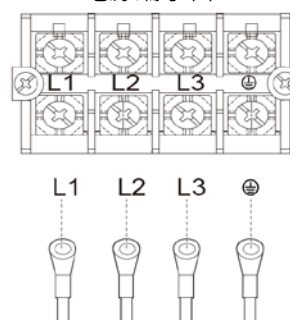
電源端子台
