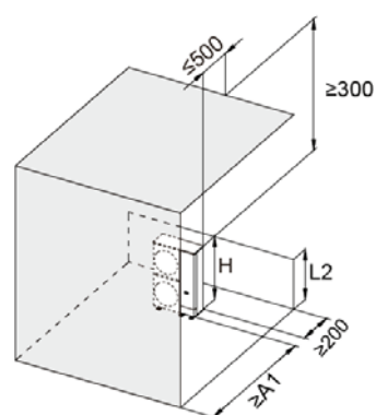
單台室外機
