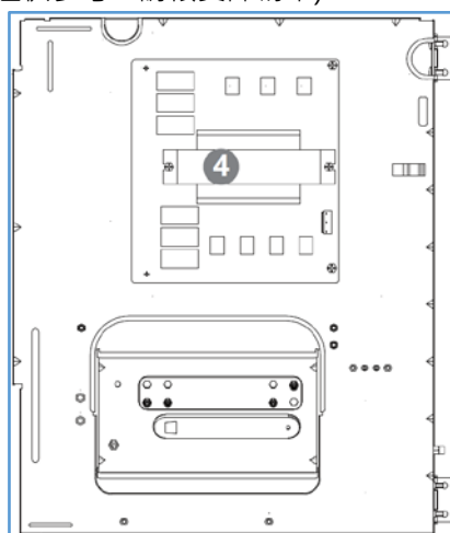
上電控箱-背面
